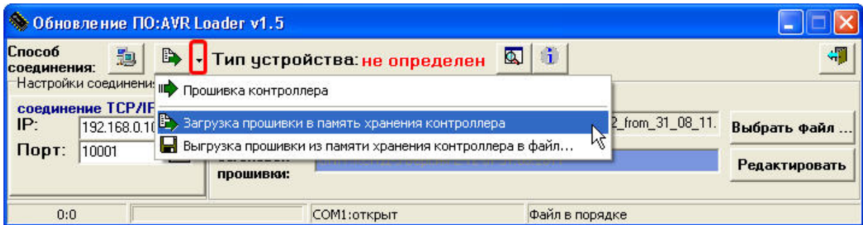
Рисунок П6.15 – Выбор режима прошивки контроллера
