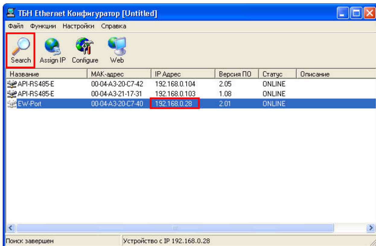
Рисунок ПЗ.3. Окно с найденными в сети устройствами
