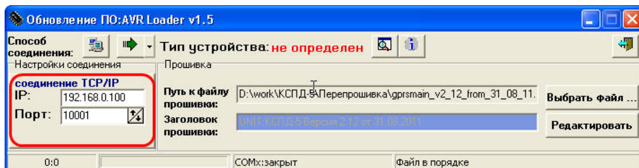
Рисунок П6.14 – Пользовательский интерфейс для режима удаленного обновления ПО через TCP/IP
