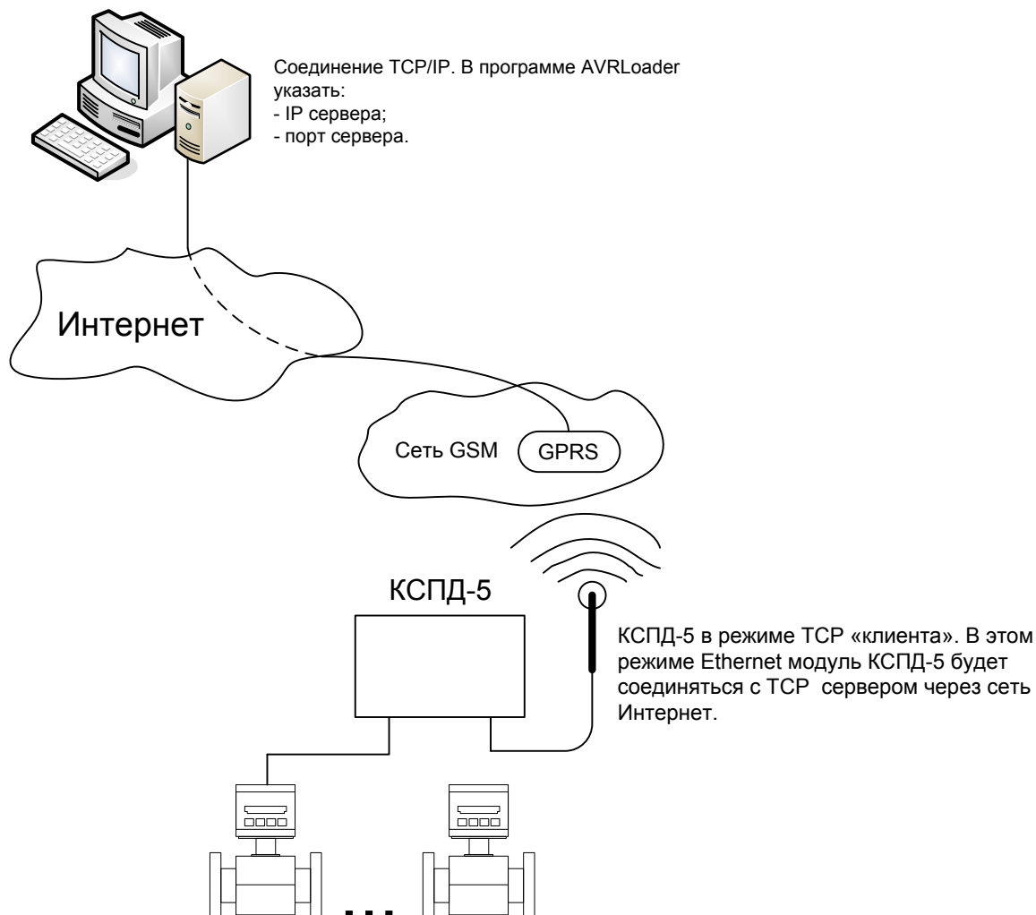
Рисунок П6.13 — Удаленное обновление ПО КСПД-5 через соединение TCP/IP
