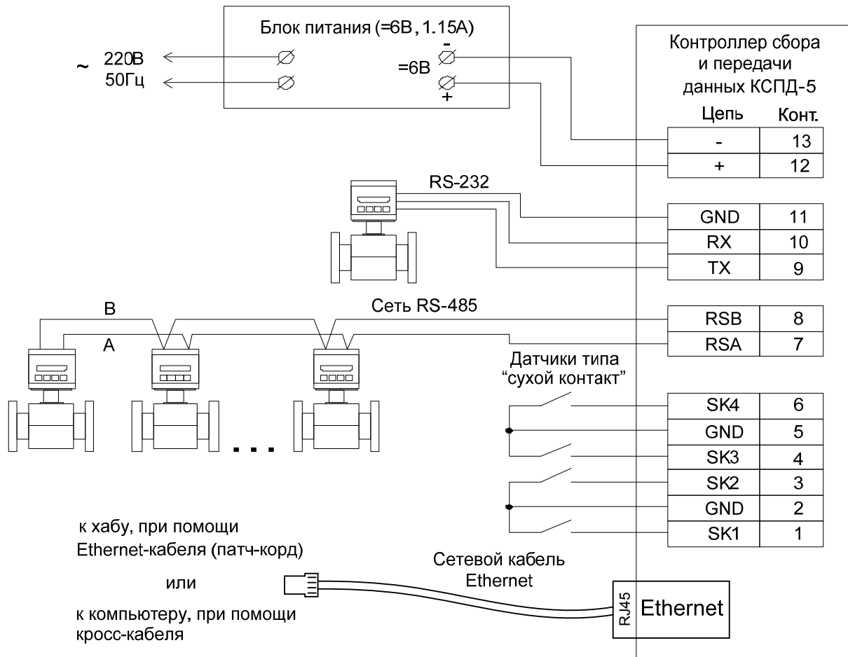
Рисунок П1.5 — Пример подключения Ethernet-модуля к плате КСПД-5
