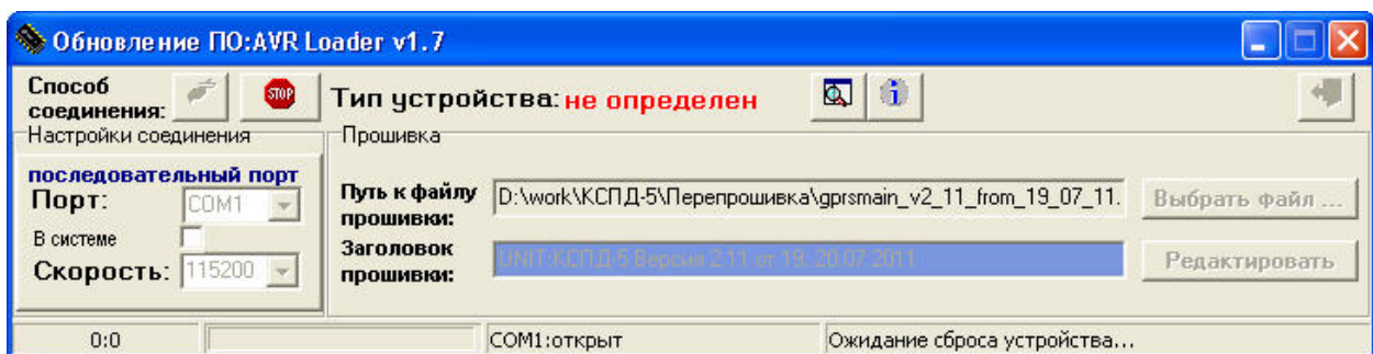
Рисунок П6.4 — Программа загрузки ожидает готовности контроллера к загрузке обновления
