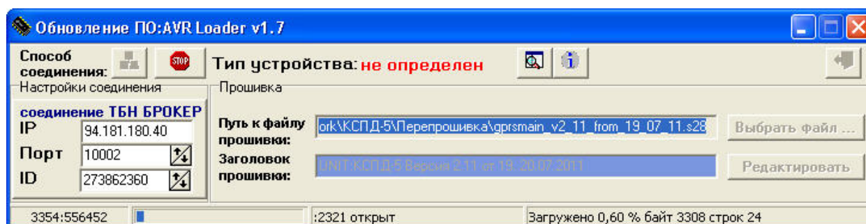
Рисунок П 6.11 – Программа ведет загрузку обновления в контроллер
