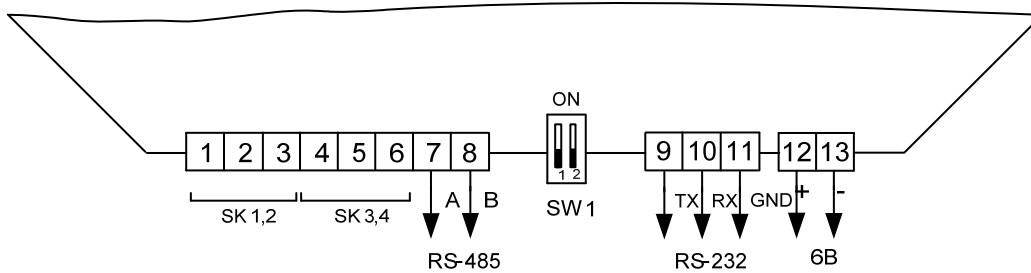
Рисунок П1.2 — Расположение переключателя SW1 на плате КСПД-5
