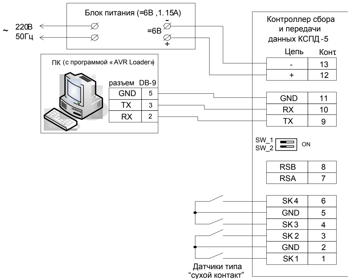
Рисунок П 6.1 — Пример подключения ПК (с программой «AVR Loader») к плате КСПД-5
