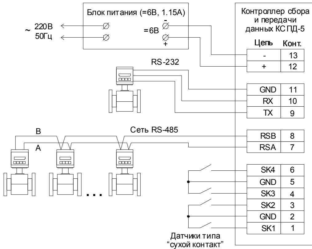
Рисунок П1.1 — Монтаж электрических цепей
