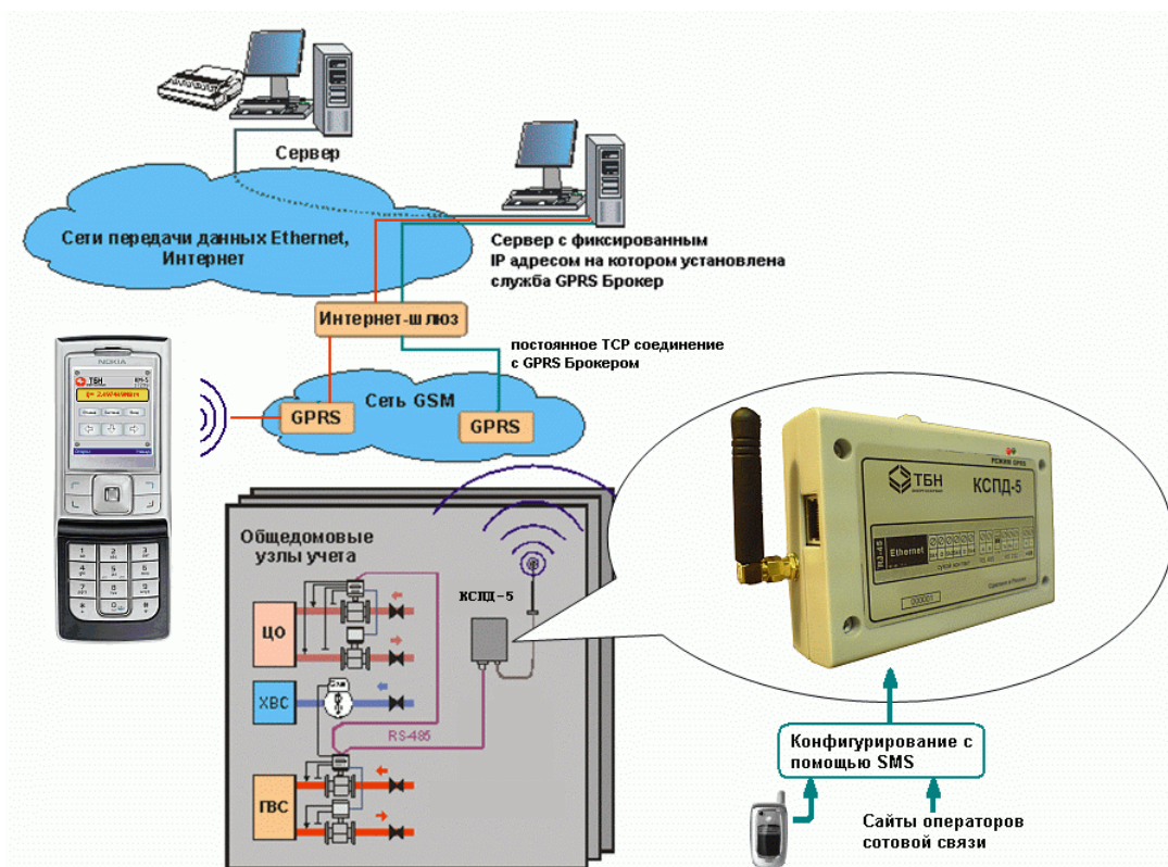
Рисунок 1 — Общая схема передачи данных по каналу GPRS
