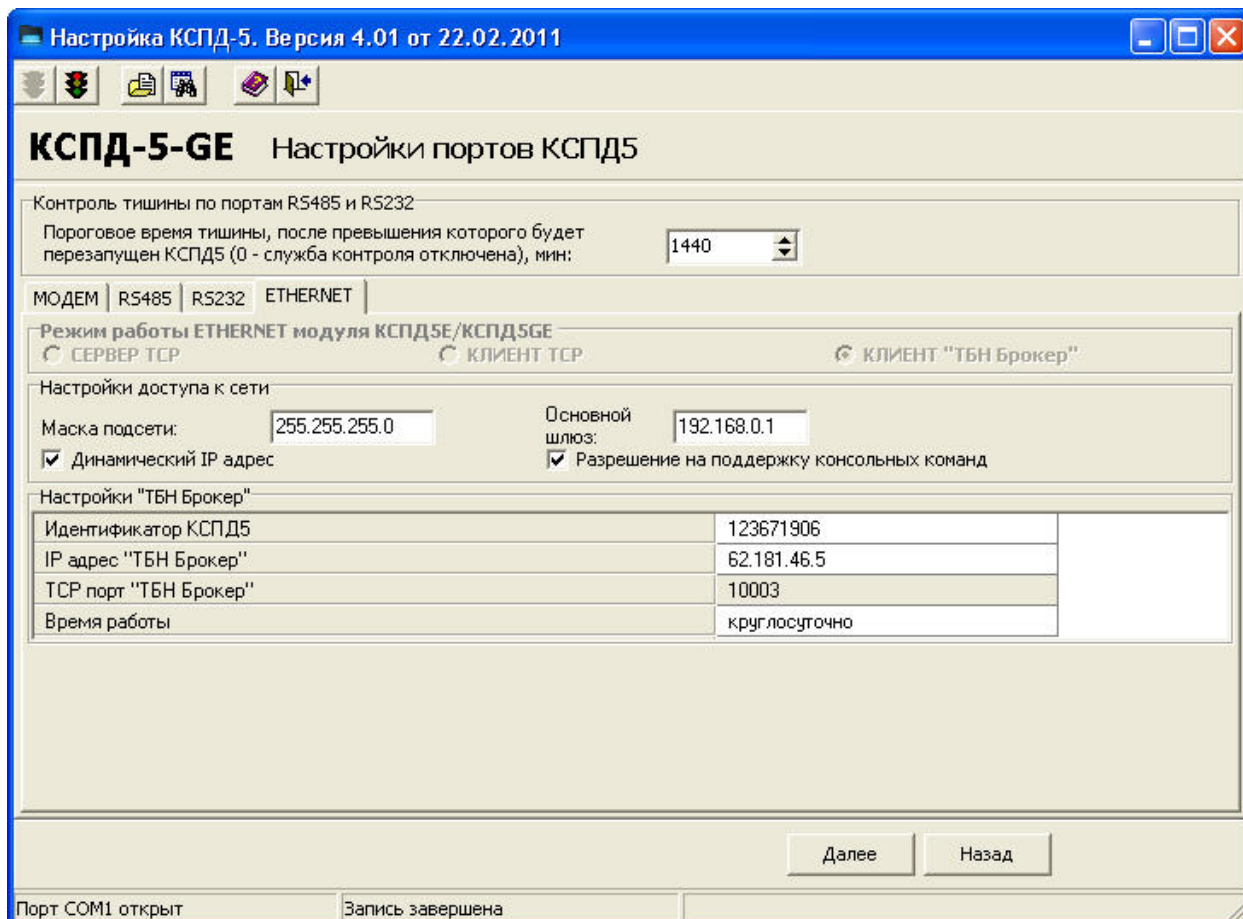
Рисунок П3.1. Окно настройки Ethernet-модуля с помощью программы «Настройка КСПД-5».
