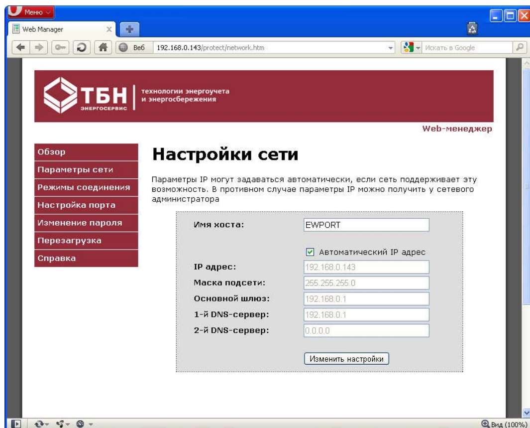
Рисунок ПЗ.5. Окно WEB-интерфейса, страница Параметры сети
