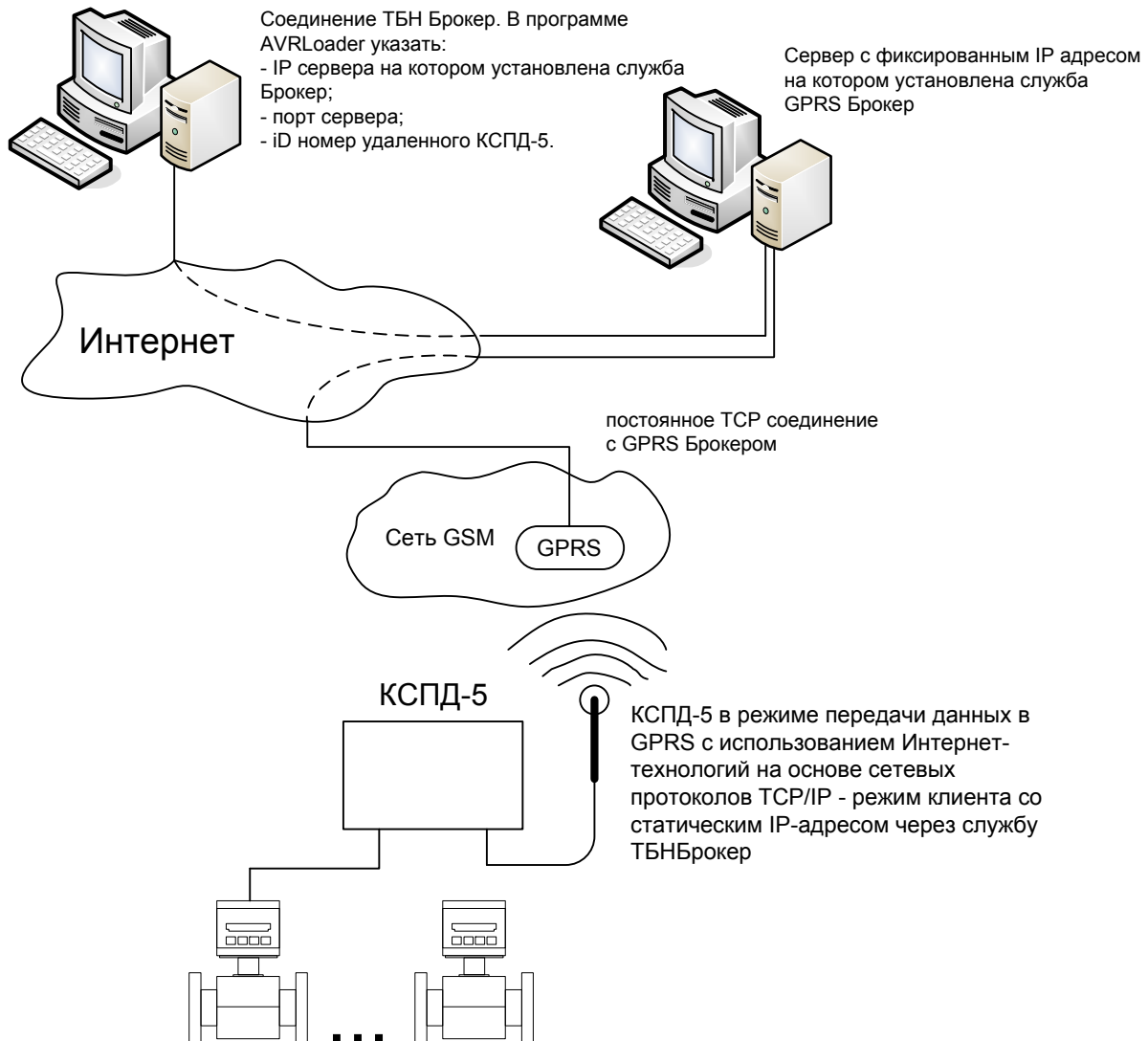
Рисунок П 6.8 — Удаленное обновление ПО КСПД-5 через соединение с ТБНБрокером
