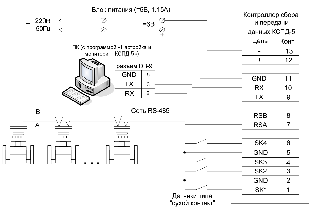
Рисунок П1.4 — Пример подключения ПК (с программой «Настройка КСПД-5») к плате КСПД-5
